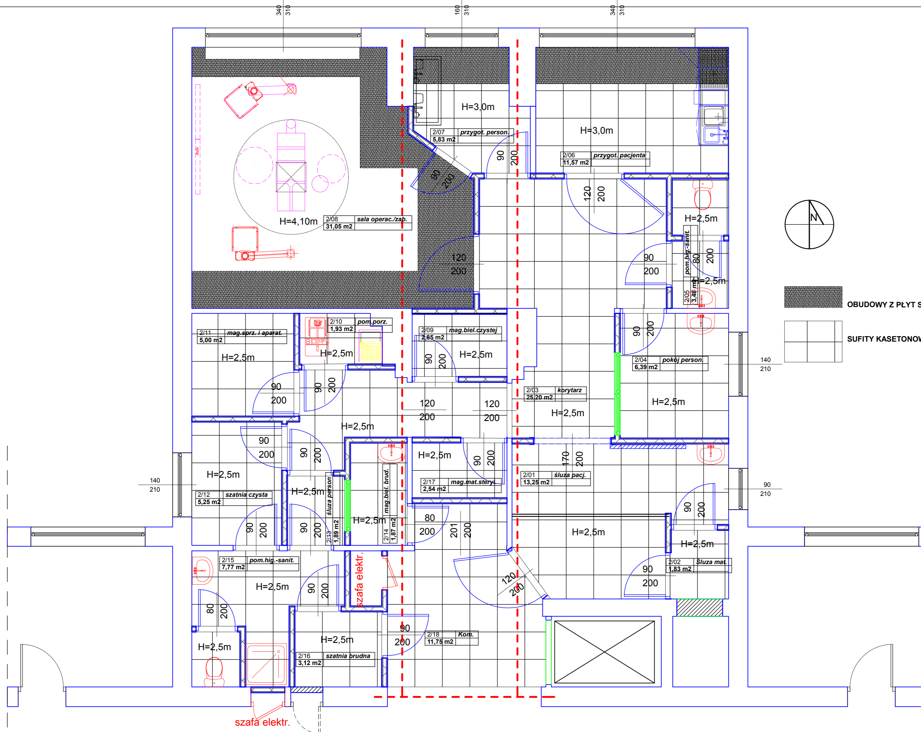
Blok operacyjny (1 sala operacyjno-zabiegowa)
